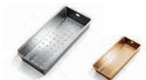
Odkapní miska - nerezová ocel 420 x 190 x 72 mm
